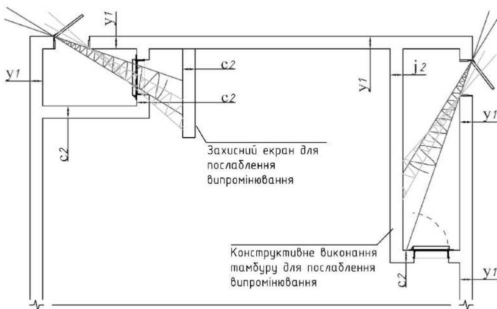
Рисунок Г.2.3 – Приклад можливого варіанту конструктивного виконання огорожувальних конструкцій вхідного тамбуру та захисного екрану
